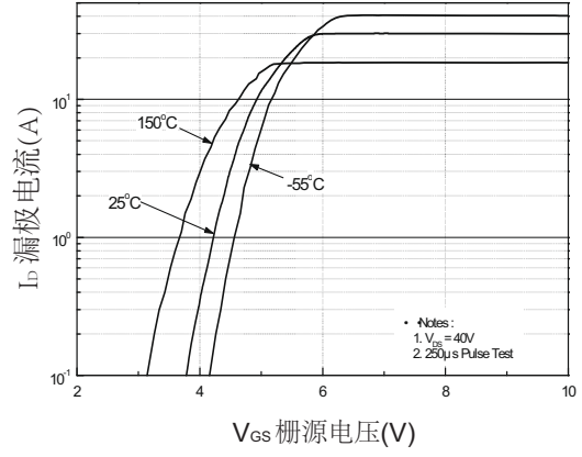
图2. 变化特性
