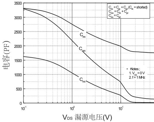
图5. 电容特性
