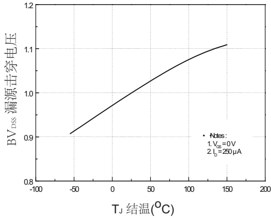
图7. 击穿电压与温度的关系
