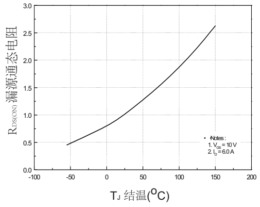
图8. 通态电阻与温度的关系
