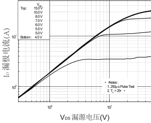
图1. 导通特性
